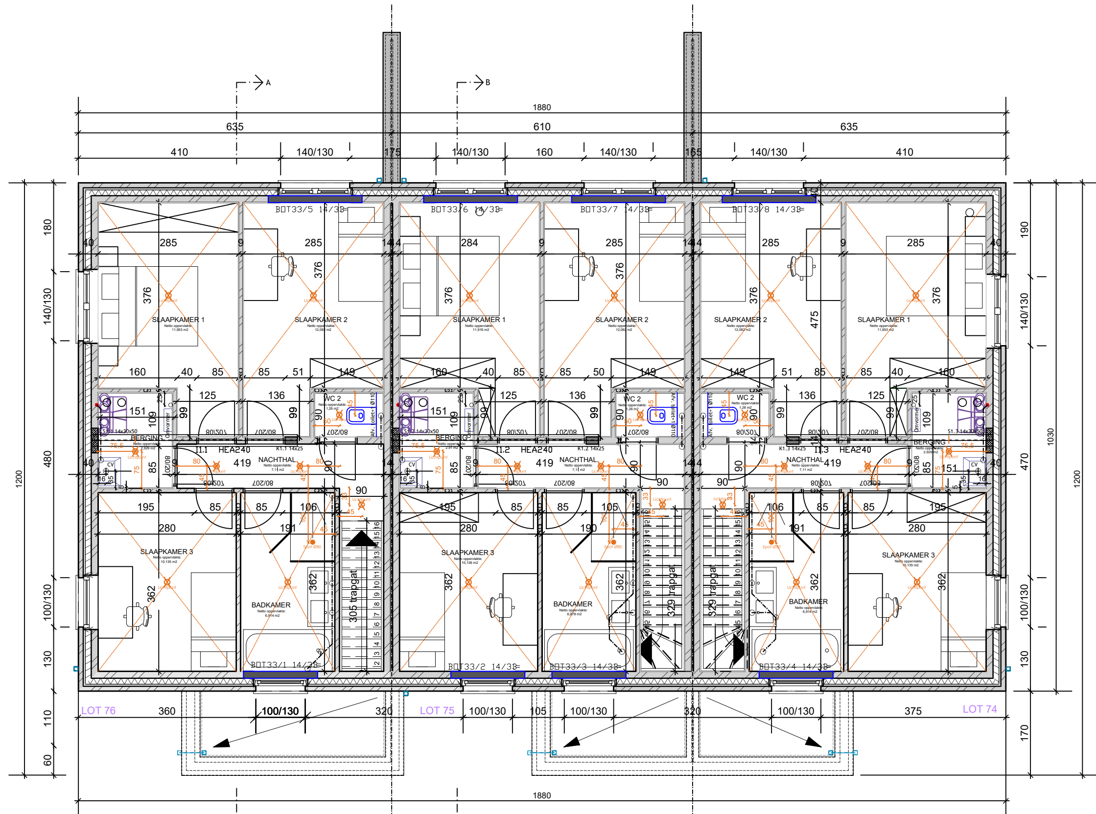
VERDIEPINGSPLAN
